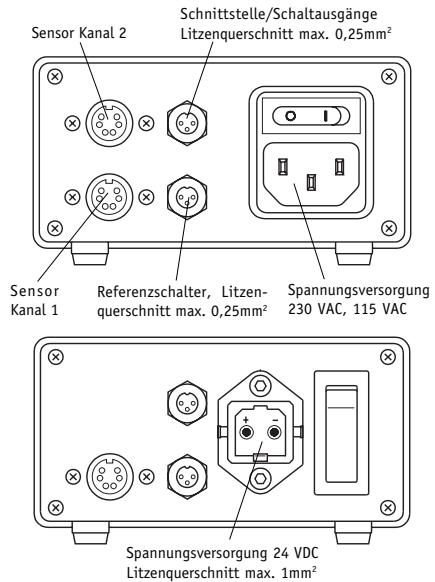
Abb. 3: Anschlussbelegung TG
