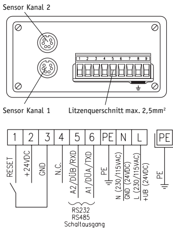
Abb. 2: Anschlussbelegung EG
