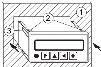
Abb. 1: Einbau
