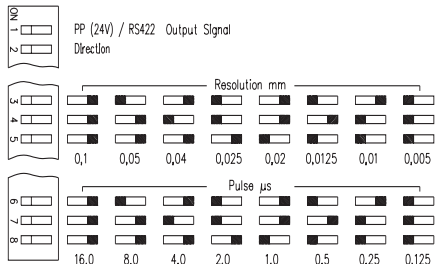
Abb. 2: DIP-Schalter-Einstellungen
