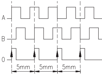
Abb. 3: Ausgangssignale A und B mit Referenzsignal (1 Inkrement)
