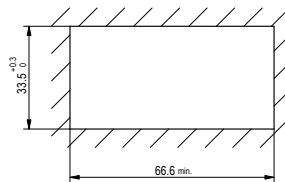
Abb. 1: Schalttafeleinbau
