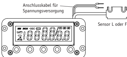
Abb. 8: Einbausatz ES
