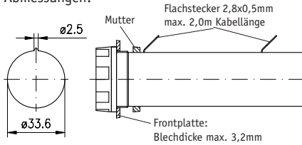
Abb. 7: Batteriehalterung
