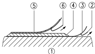
Abb. 1: Montage Magnetband
