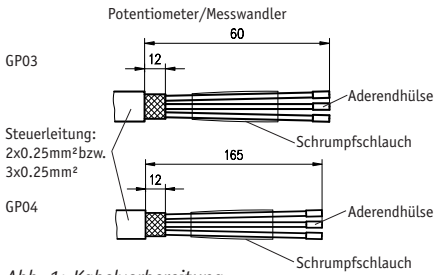
Abb. 1: Kabelvorbereitung
