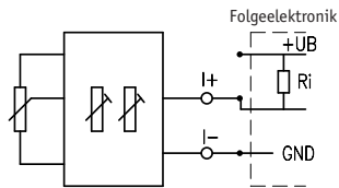
Abb. 7: Anschluss Bürde gegen +UB
