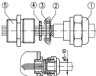
Abb. 3: Kabelanschluss PG9
