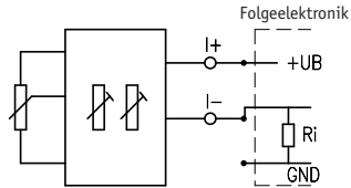
Abb. 6: Anschluss Bürde gegen Masse
