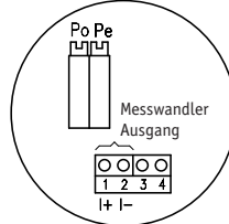
Abb. 5: Anschlussbelegung mit Messwandler
