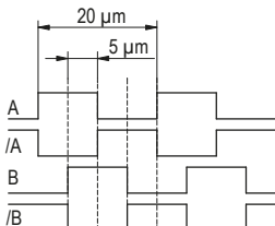
Abb. 2: Ausgabe der Quadratursignale
