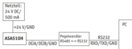
Abb. 3: Blockschaltbild RS485-Verbindung
