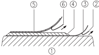
Abb. 1: Montage Magnetband
